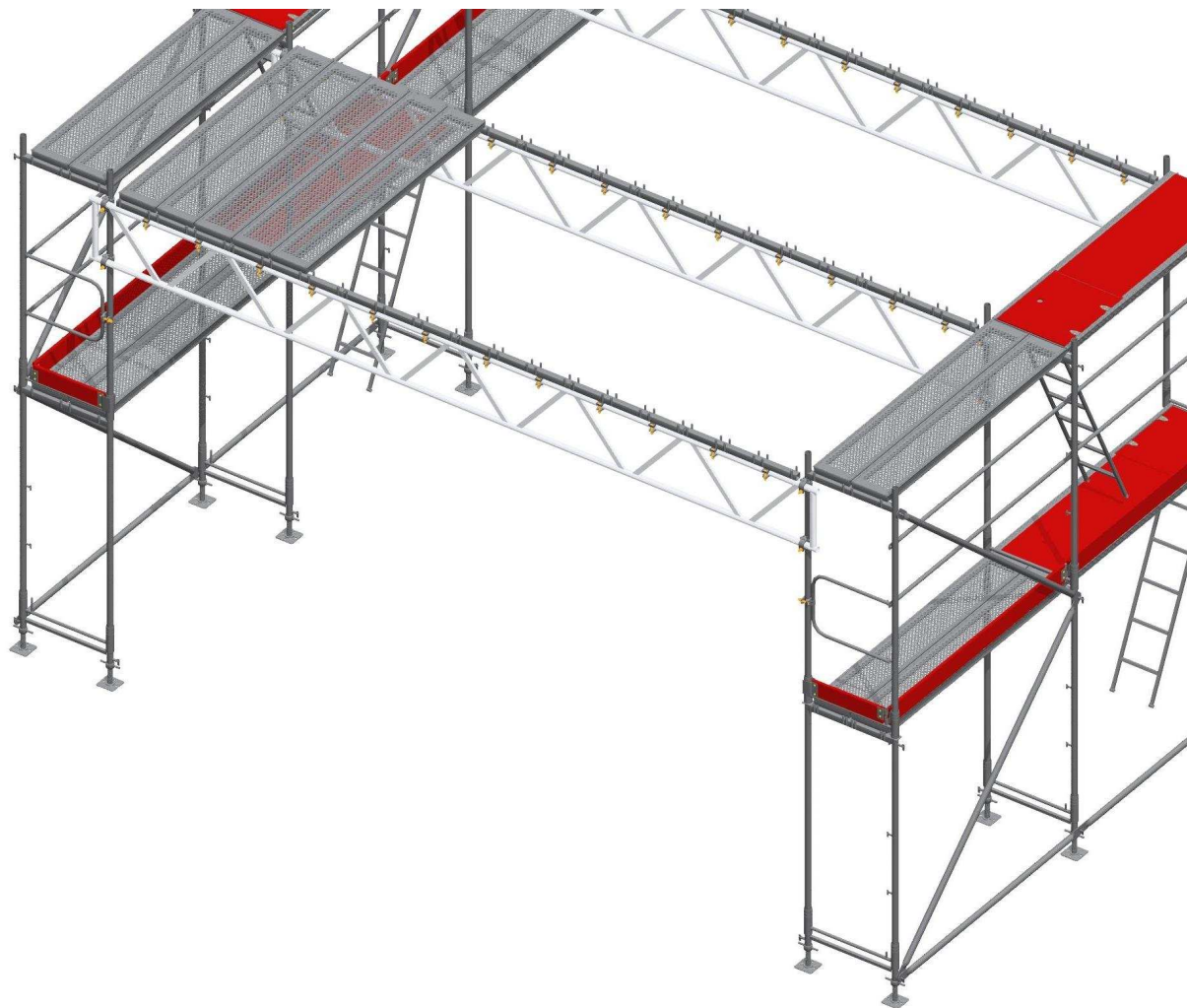
Rys. 1. Zastosowanie dźwigarów i nakładek do wykonania platformy
